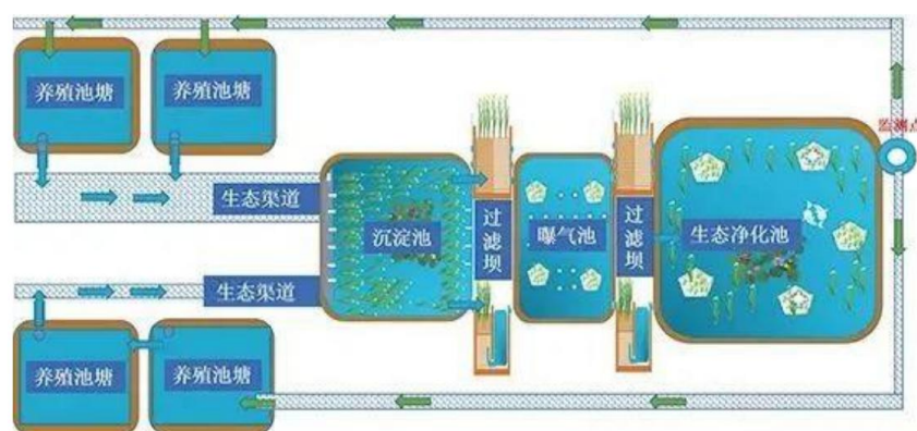
图 2-2 生态净化区工艺流程示意图
