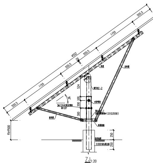
图 2-1 光伏支架结构示意图（仅供参考示意）
