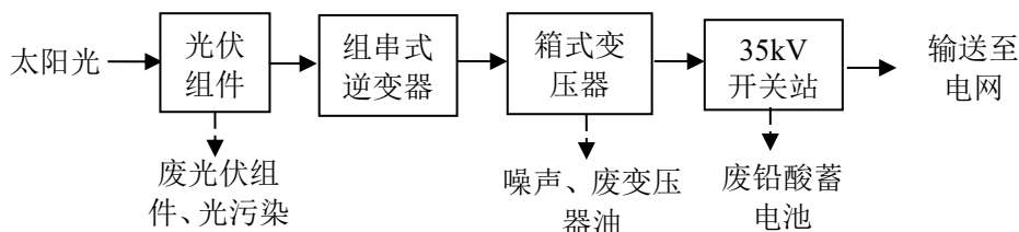
图 4-1 项目运营期工艺流程及排污产点示意图
