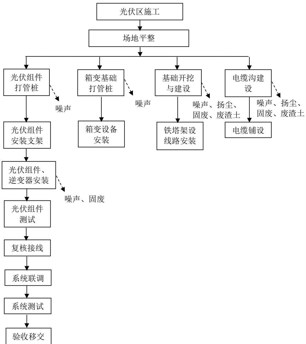
图 2-6 光伏区施工期工艺流程图
