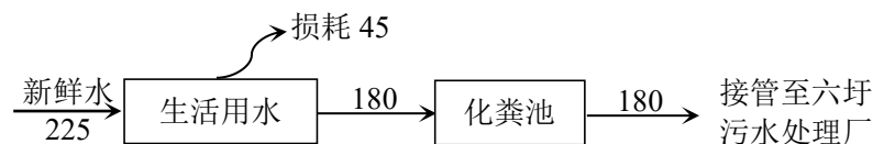
图2-1 项目水平衡图 (m³/a)
