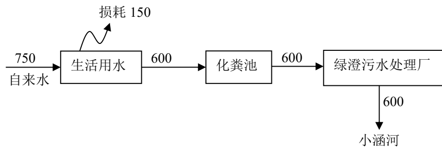
图 4-2 扩建项目水平衡图 单位: m 3 /a
