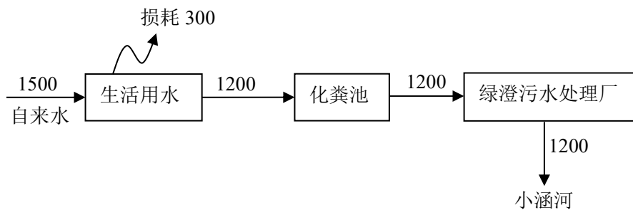
图 4-3 全厂水平衡图 单位: m 3 /a
